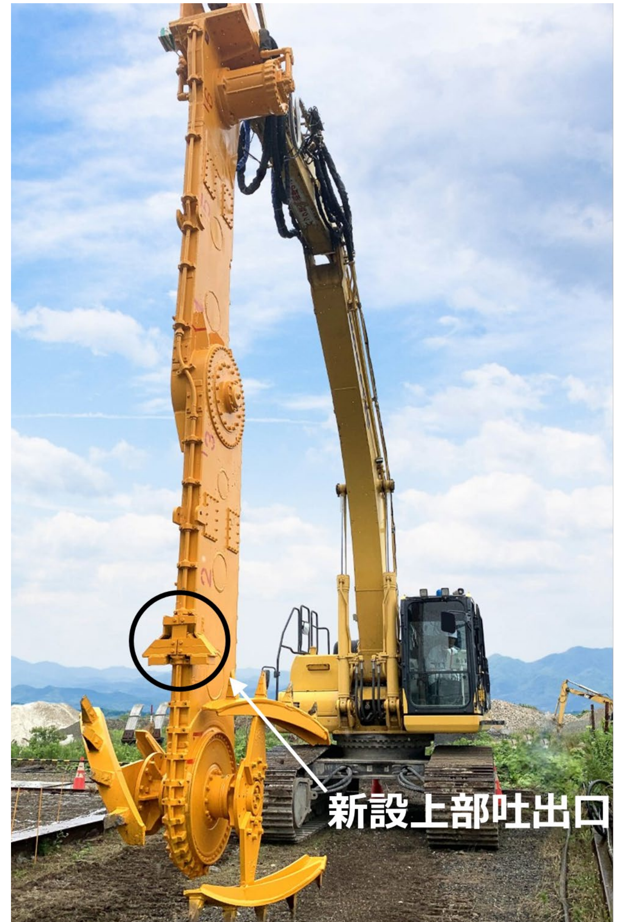
WILL-m工法施工機械全景
