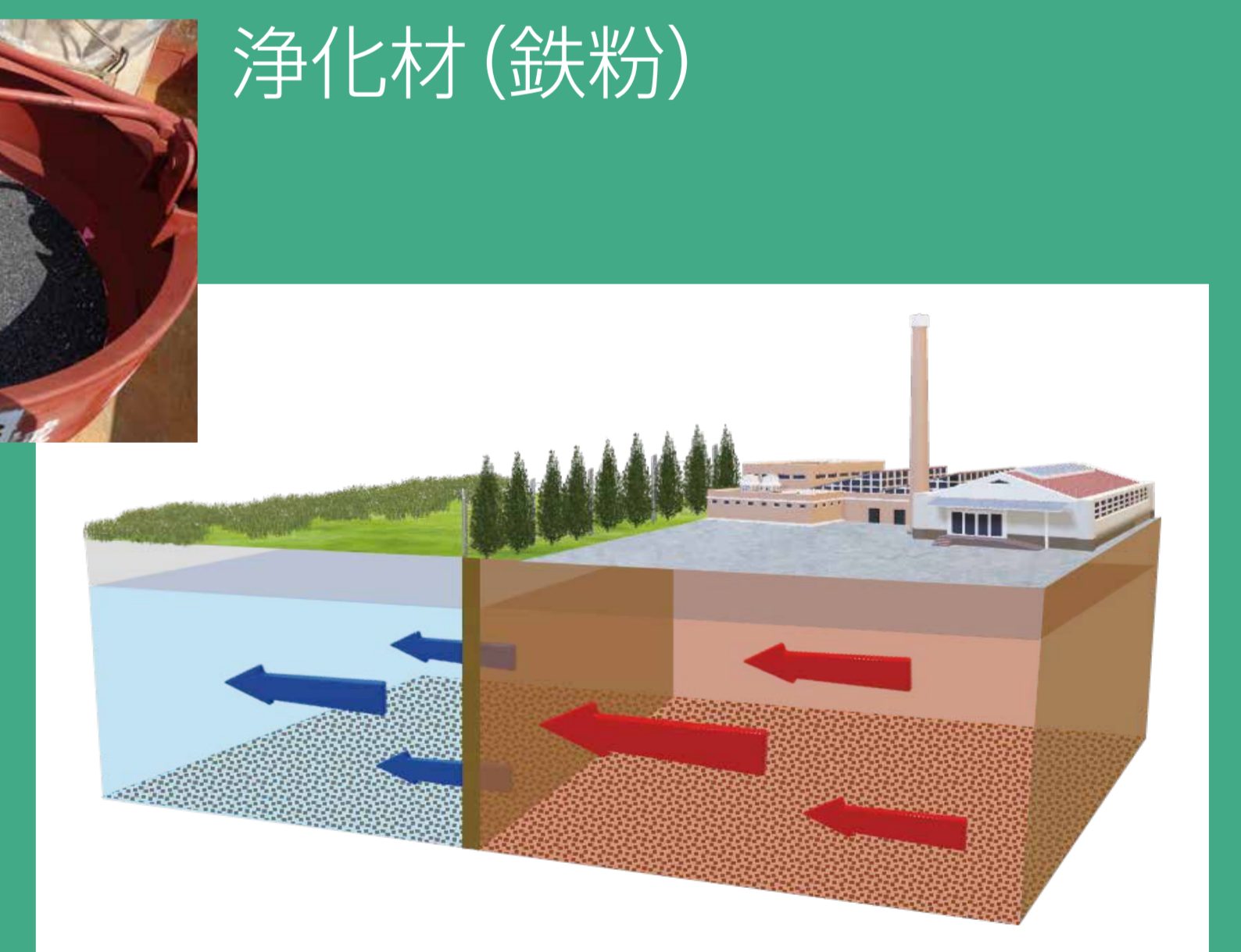
透過性浄化壁による浄化イメージ
