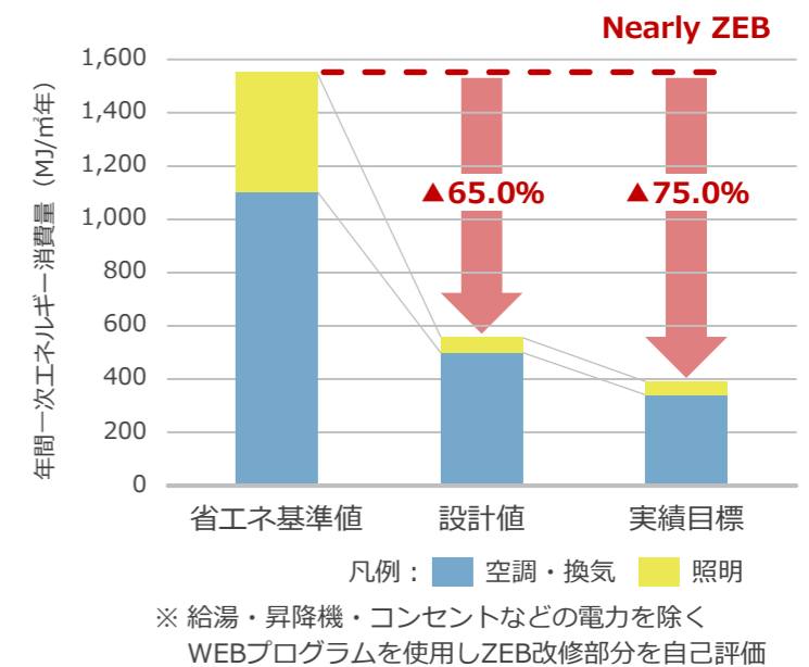
ZEB改修部分の年間一次エネルギー消費量
